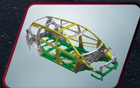
โครงสร้างตัวถัง (TECT) และระบบ NVH ถูกออกแบบจากเหล็กกล้าที่มีน้ำหนักเบาและทนทานต่อการสึกหรอเป็นพิเศษ พร้อมทั้งช่วยลดเสียงรบกวนจากภายนอก และแรงสั่นสะเทือนขณะขับขี่ เพื่อความปลอดภัยสูงสุด และนุ่มนวลตลอดการเดินทาง
