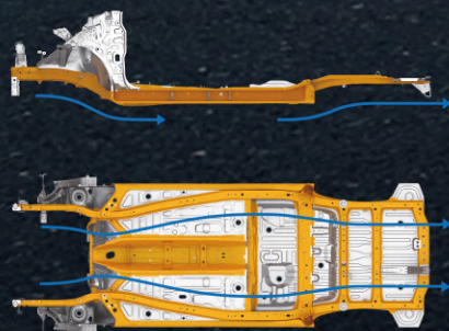
โครงสร้างช่วงล่างจากเหล็ก High-tensile เชื่อมต่อกันอย่างสมบูรณ์แบบ ให้ความแข็งแรง ปลอดภัยในทุกการขับขี่ และประหยัดน้ำมันมากขึ้น
